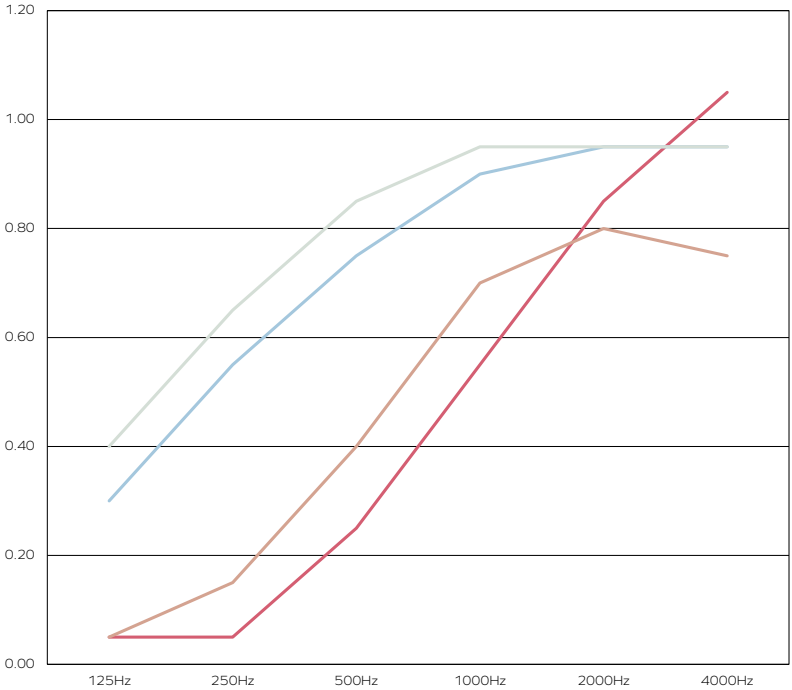
Sound Absorption Coefficient ( \alpha_s ) according to EN ISO 354 Universität Stuttgart – Institut für Akustik und Bauphysik IABP
