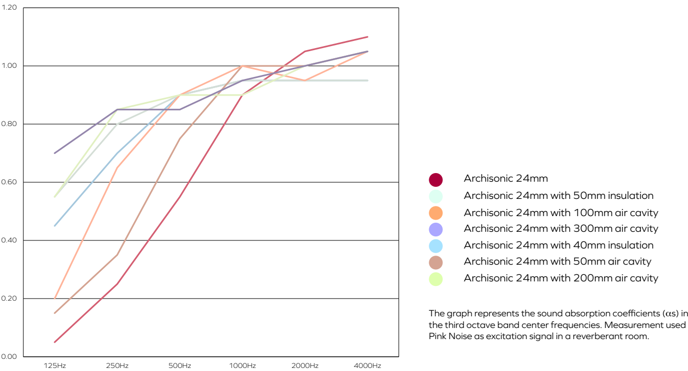
Sound Absorption Coefficient ( \alpha_s ) according to EN ISO 354 Universität Stuttgart – Institut für Akustik und Bauphysik IABP
